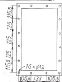
Inlet flange DIN 24 193-2
